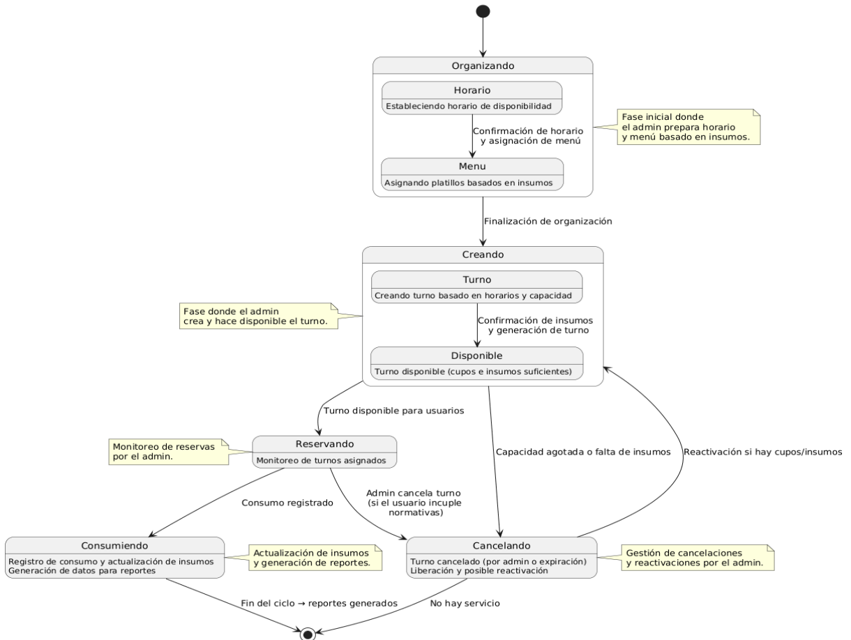
Diagrama de Estados - Acciones del Administrador Ciclo de Vida de un Turno - Gestión Comedor Universitario UCV
